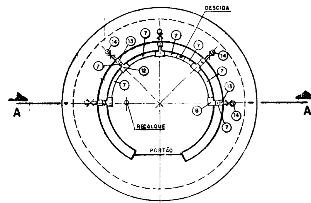
NÍVEL - 01 ESC - 1/25
