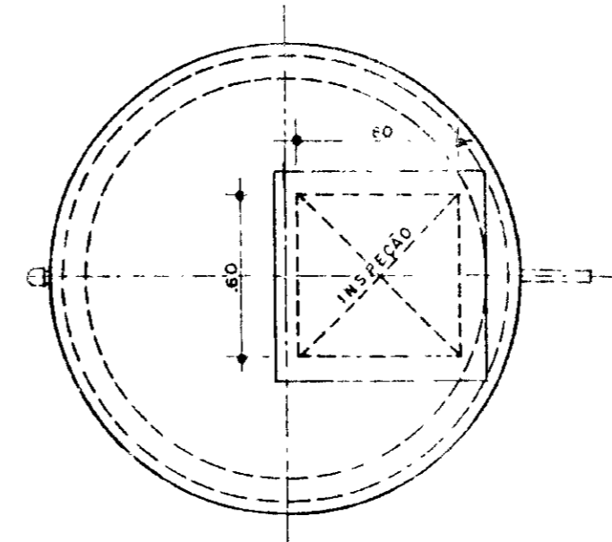
VISTA SUPERIOR ESC - 1/25
