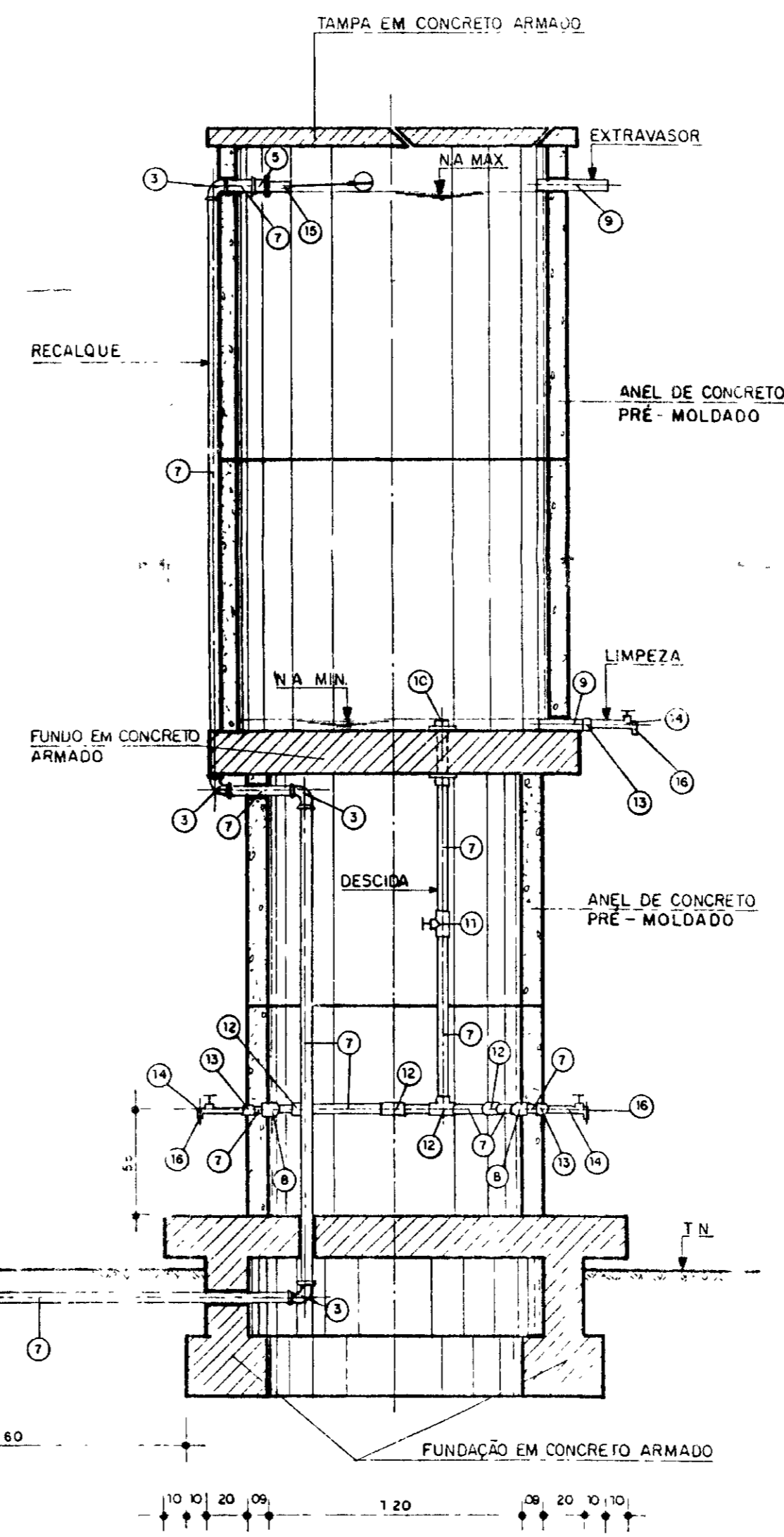
CORTE - AA ESC - 1/25
