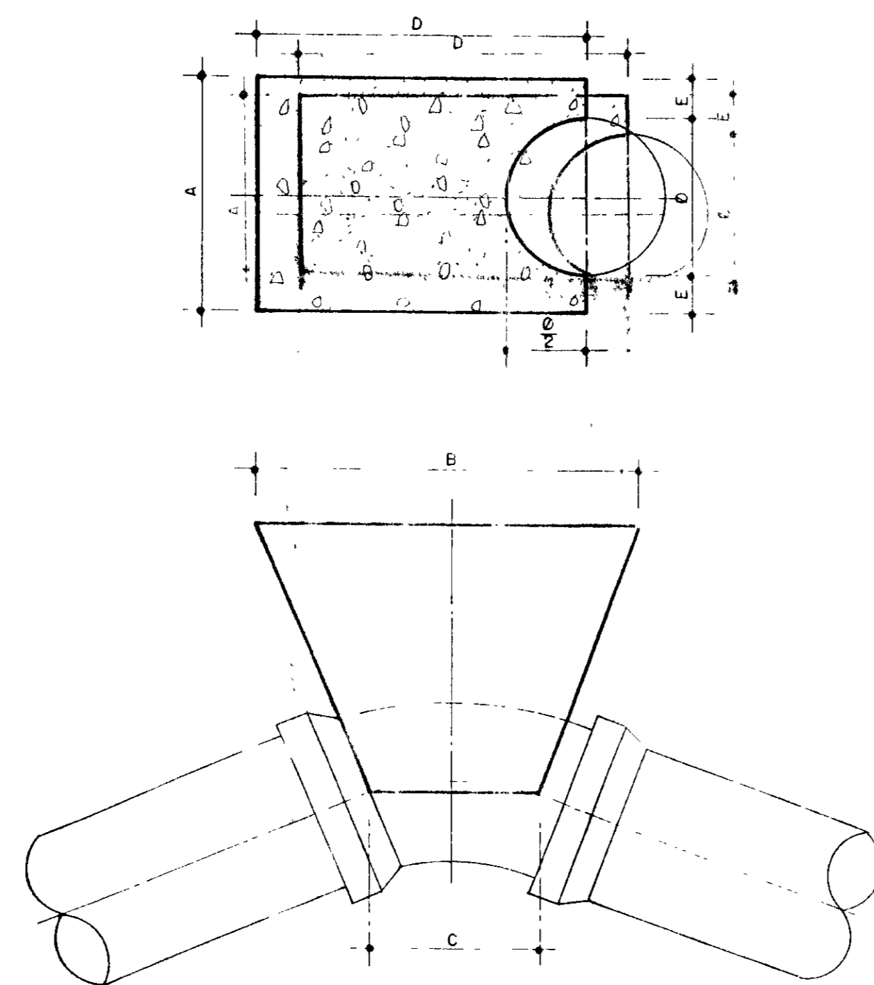
CURVA 45°
