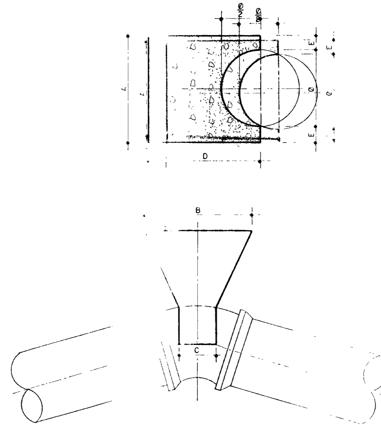
CURVA 22° 30'
