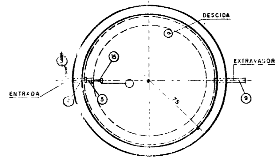
NÍVEL - 02 ESC - 1/25
