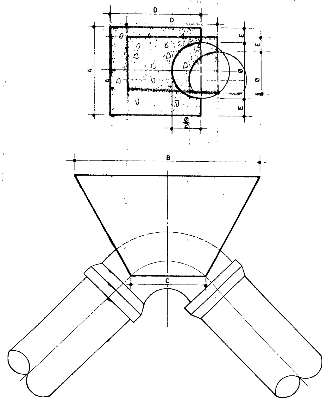
CURVA 90°
