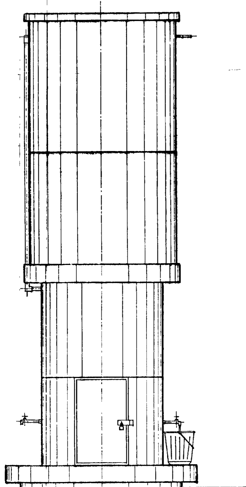
FACHADA PRINCIPAL ESC - 1/25
